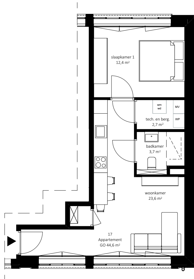
Eerste verdieping
