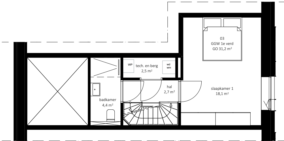
Eerste verdieping
