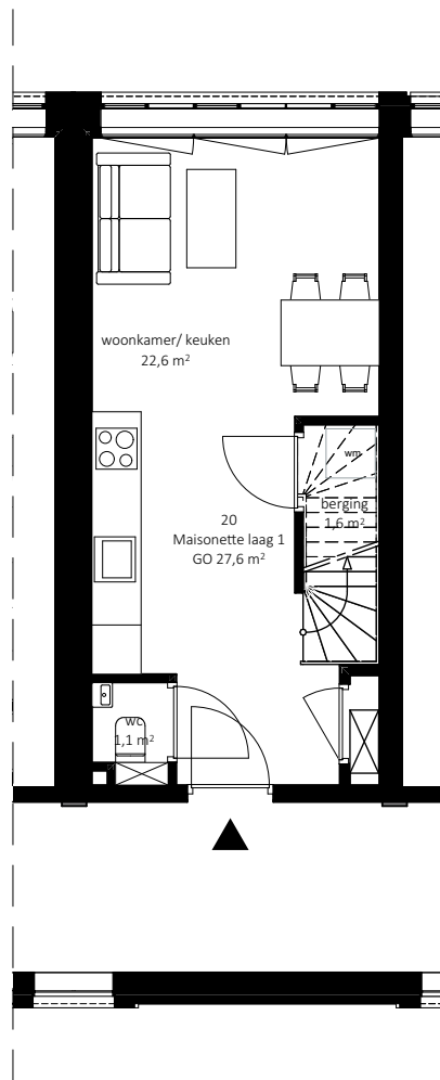
Tweede verdieping
