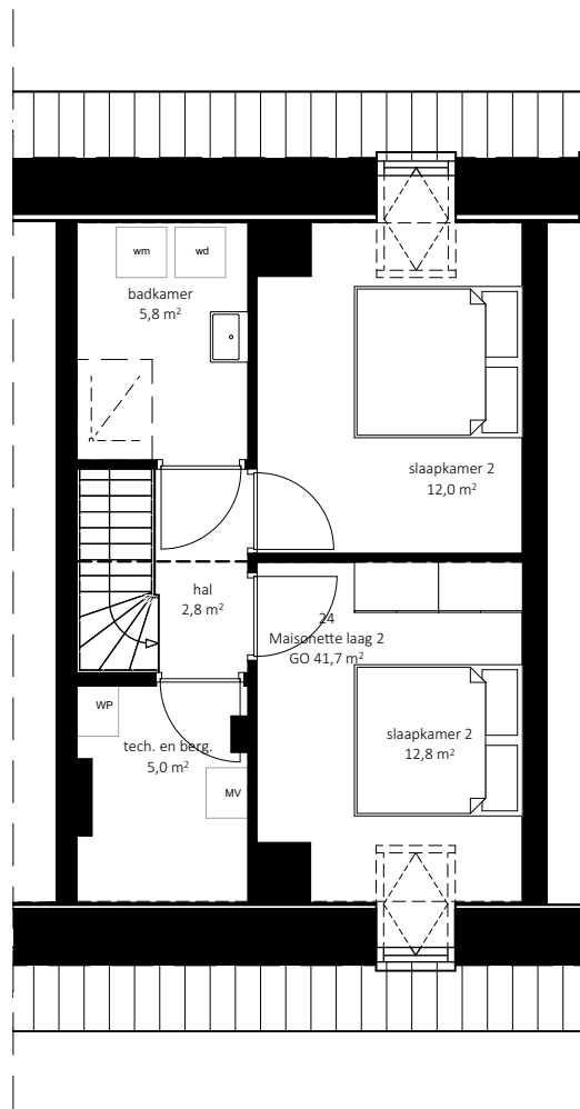
Derde verdieping
