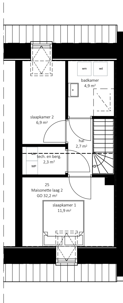
Derde verdieping
