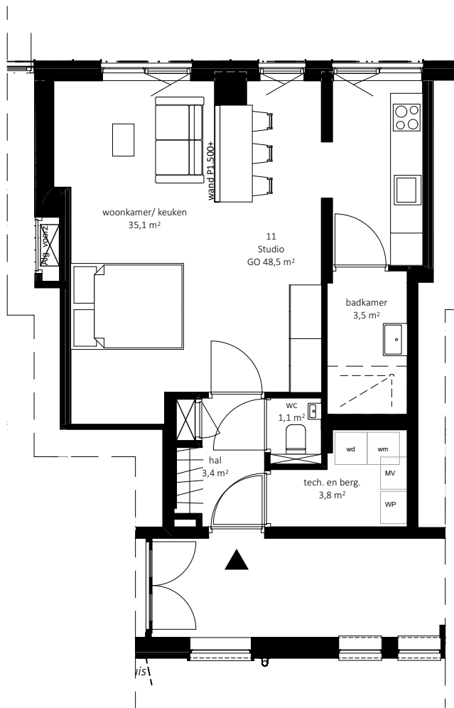
Beganegrond
