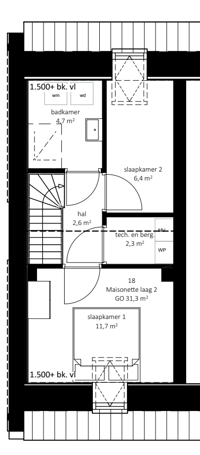
Derde verdieping
