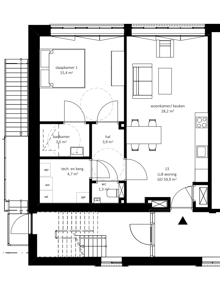
Eerste verdieping
