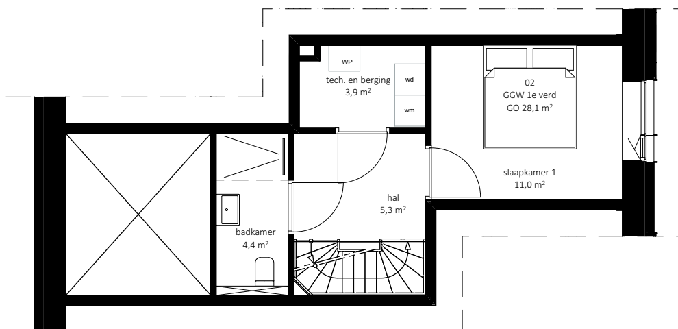
Eerste verdieping
