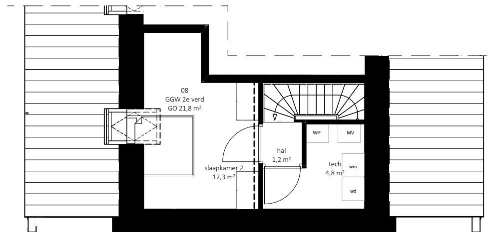
Tweede verdieping
