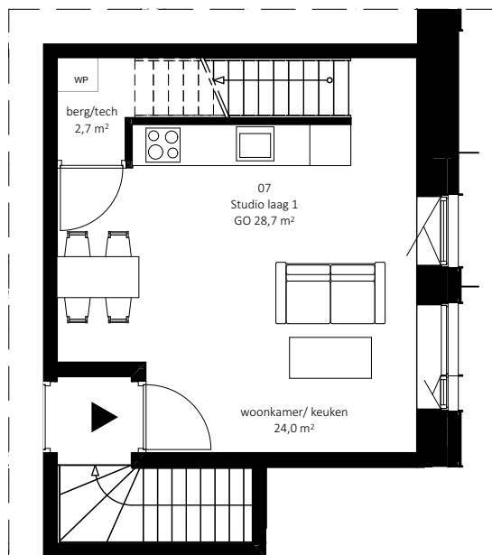
Eerste verdieping
