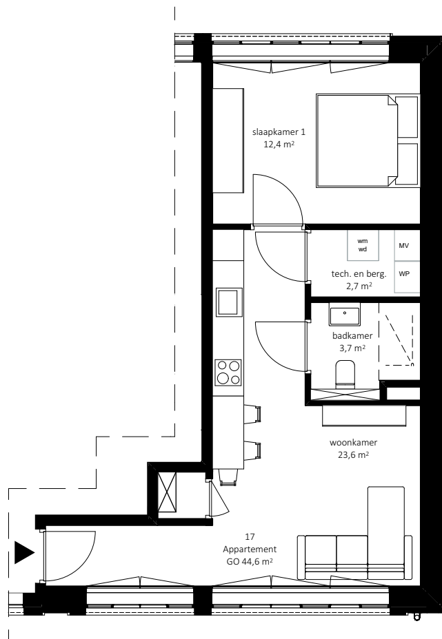
Eerste verdieping
