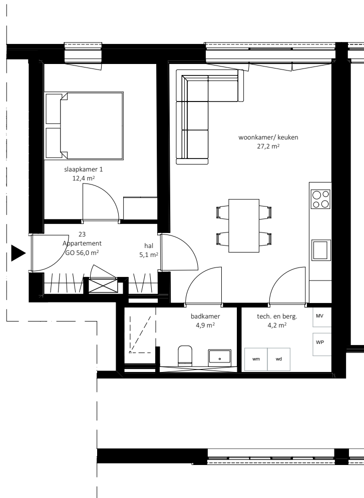
Eerste verdieping
