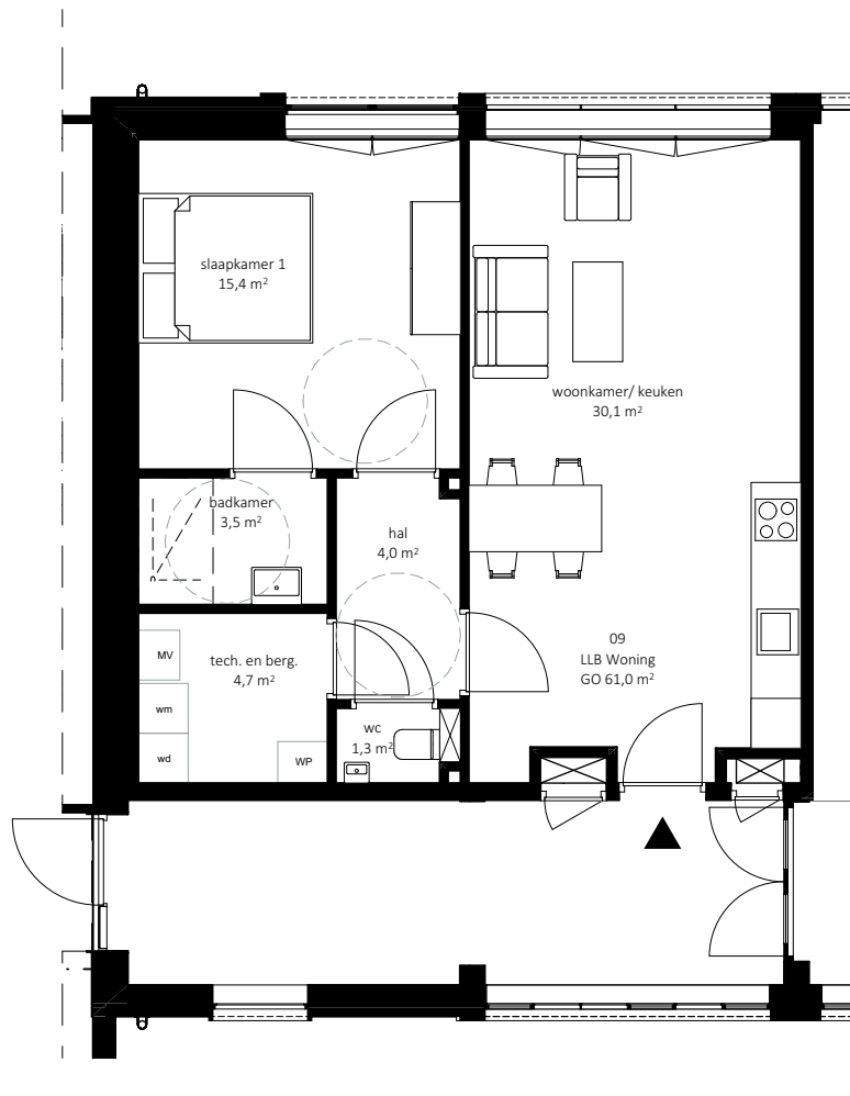
Beganegrond
