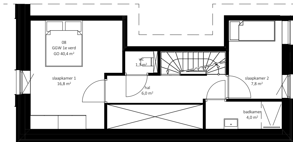
Eerste verdieping
