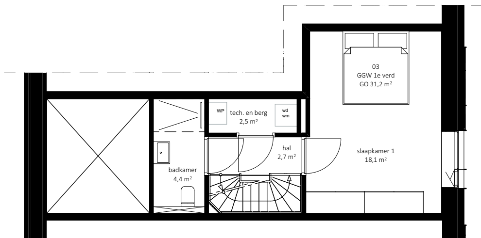
Eerste verdieping
