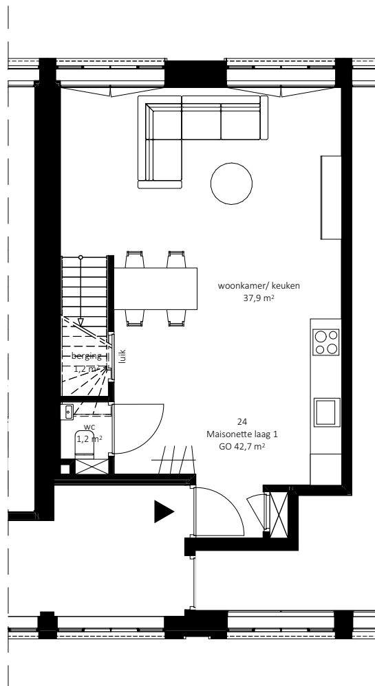
Tweede verdieping
