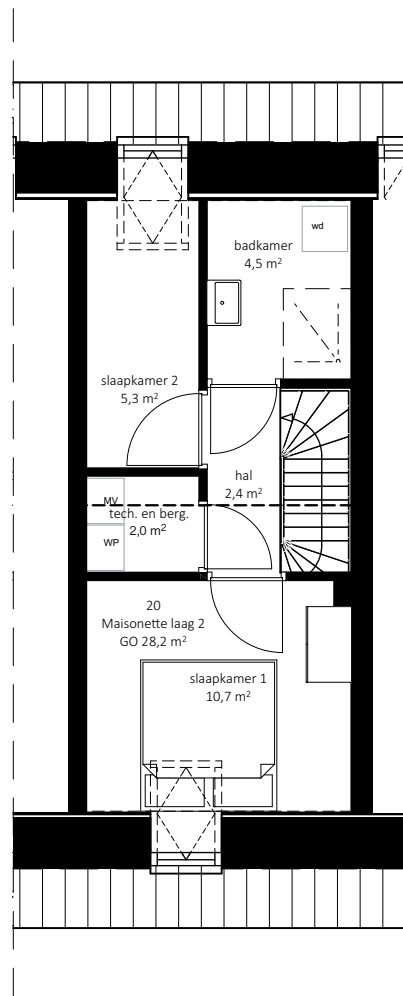
Derde verdieping
