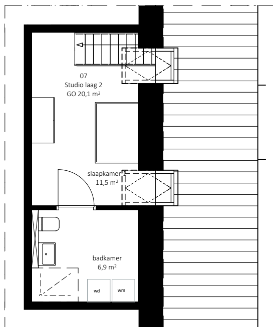
Tweede verdieping
