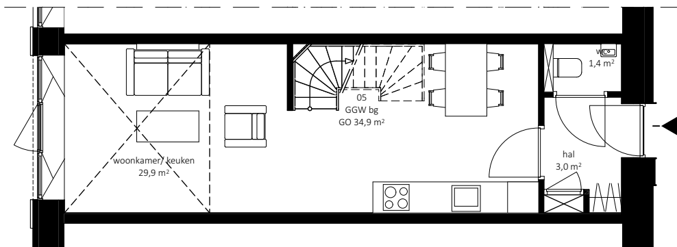
Begane grond
