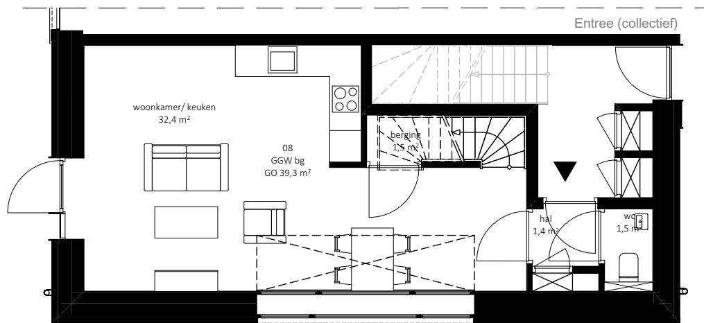
Begane grond
