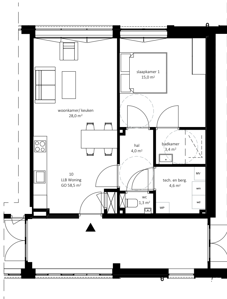
Beganegrond
