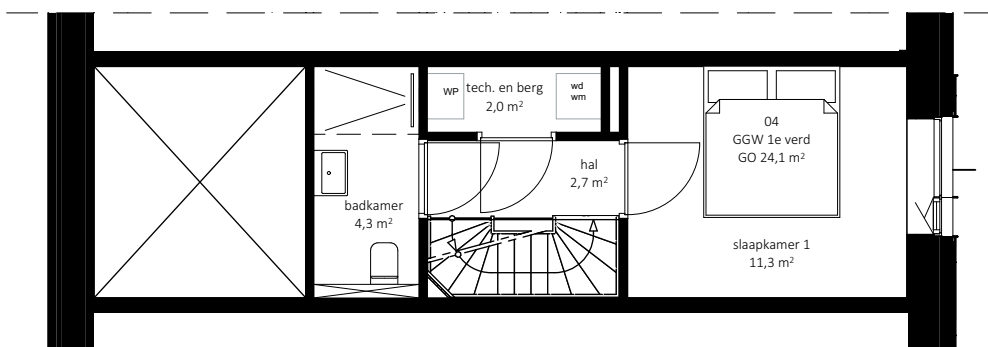
Eerste verdieping
