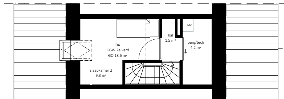
Tweede verdieping
