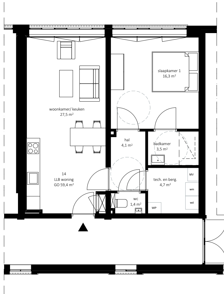
Eerste verdieping
