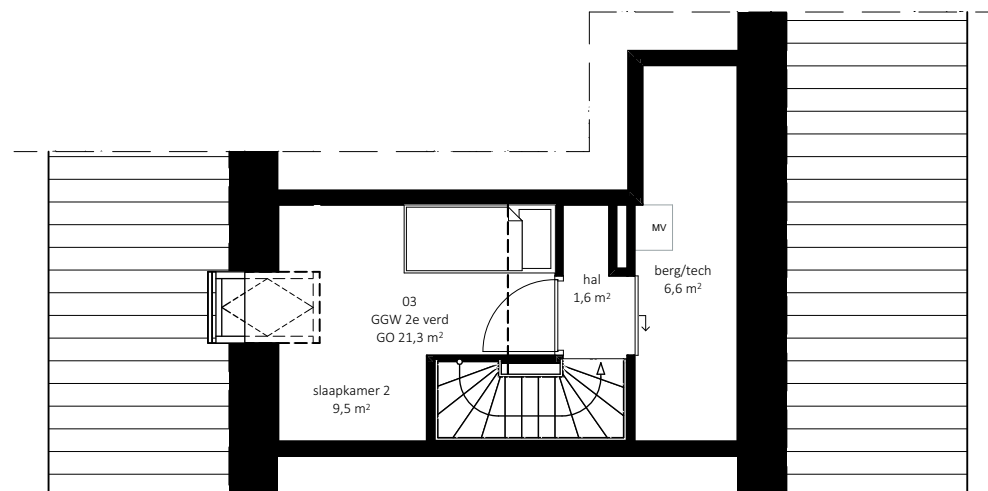
Tweede verdieping
