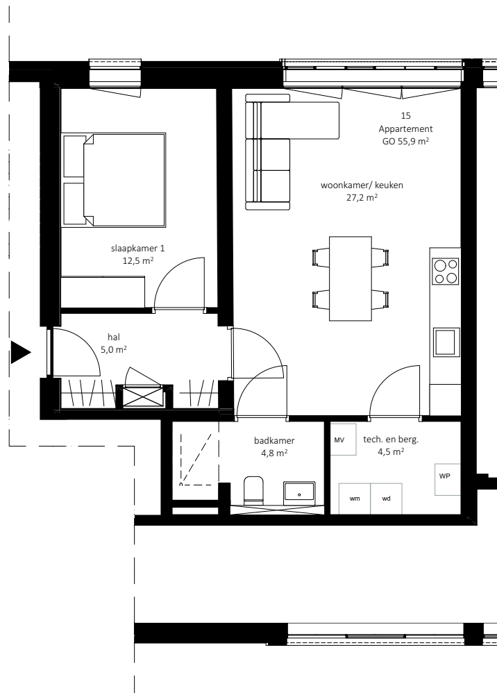
Eerste verdieping
