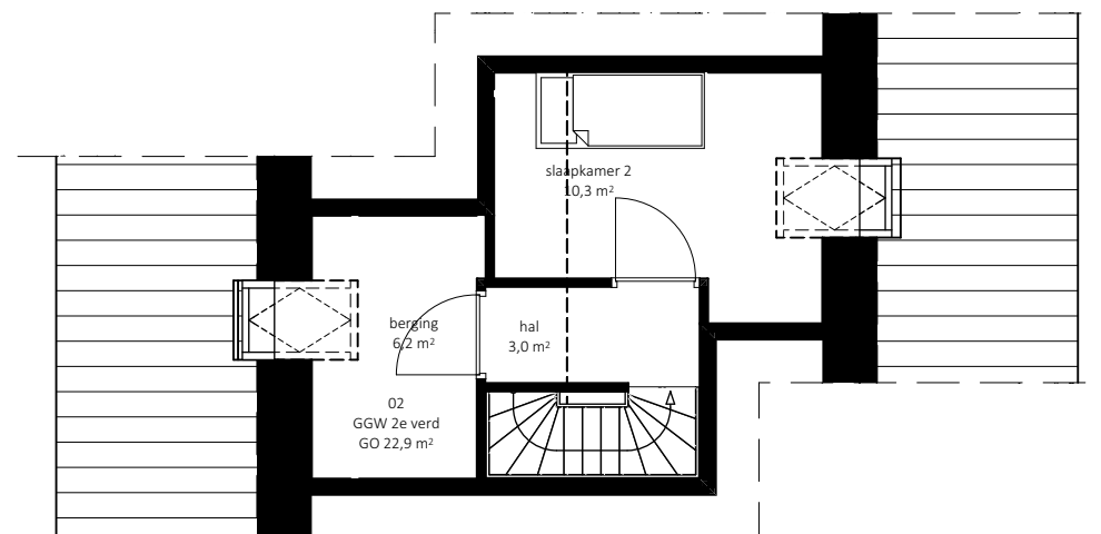
Tweede verdieping
