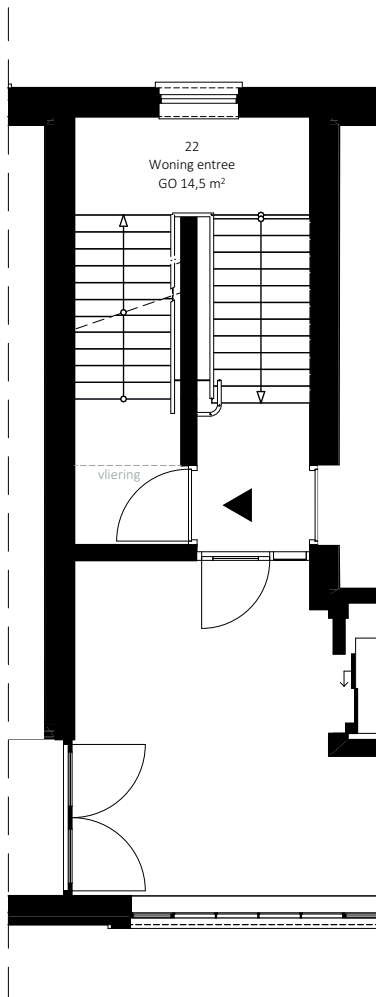
Tweede verdieping
